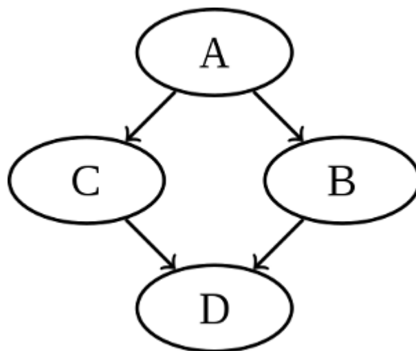
Fig. 2: Diamond DAG
