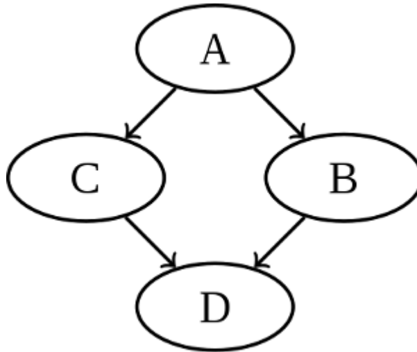
Fig. 2: Diamond DAG
